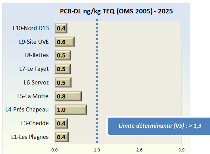
Résultats des PCB-DL dans les lichens (ng/kg TEQ OMS 2005)
