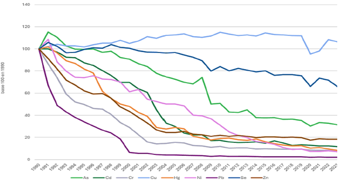
Evolution des émissions de métaux lourds entre 1990 et 2023 (base 100 en 1990)
