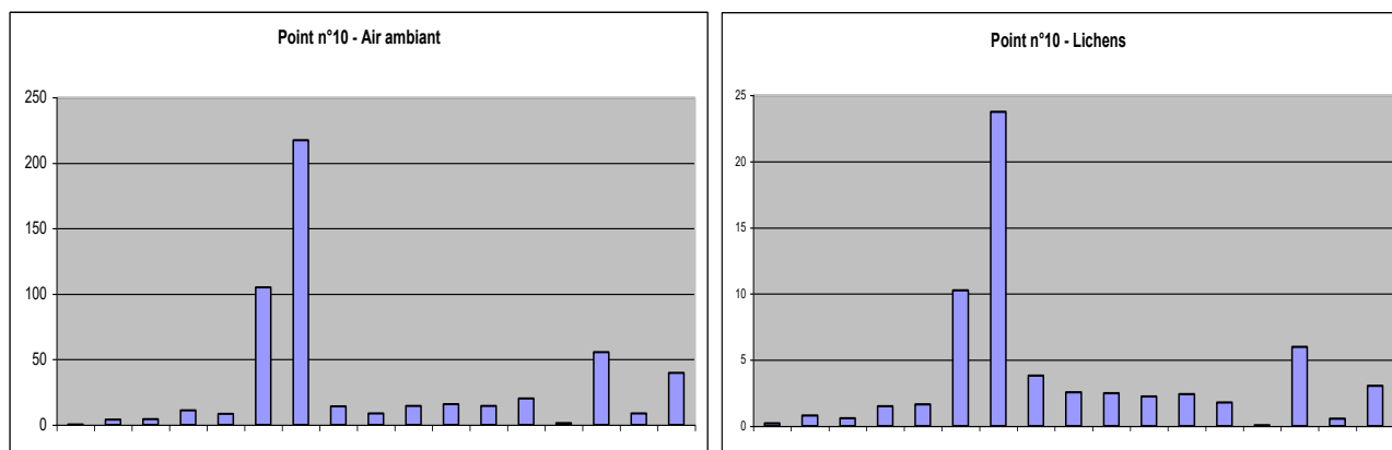
Graphique du profil de répartition des PCDD/F dans l'air ambiant et graphique du profil de répartition des PCDD/F dans les lichens sur le même site (ADEMDIOX, participation Air Lichens, 2000).
